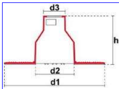
větrací komínek 1105
