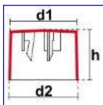
krytka 1108PK
