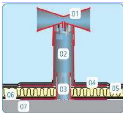
instalace komínku 1106
