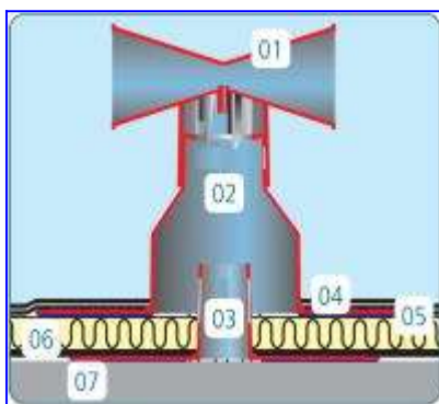
instalace komínku 1105
