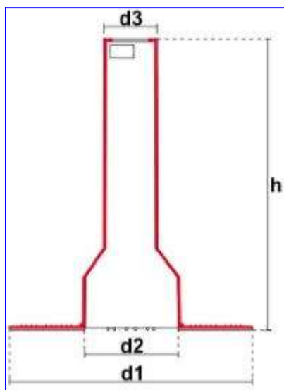
větrací komínek 1107
