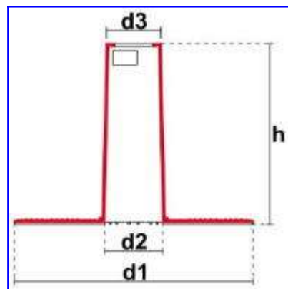
větrací komínek 1106
