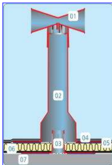
instalace komínku 1107
