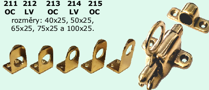
protikusy A sklapka 605 LV protikus B Výška otvoru v protikusech A: 10, 15, 20, 25 a 30 mm
