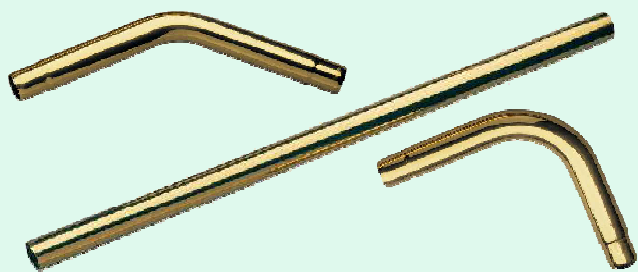
Zábradlová trubka průměr 30 nebo 35 mm rovná 150, 200, 250, 300 mm, zahnutá 90° jen 30 mm, zahnutá 135°
