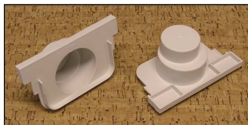
žlábek PEGASUS PLUS se nyní vyrábí v rozměru 130 x 75 x 1000 mm
