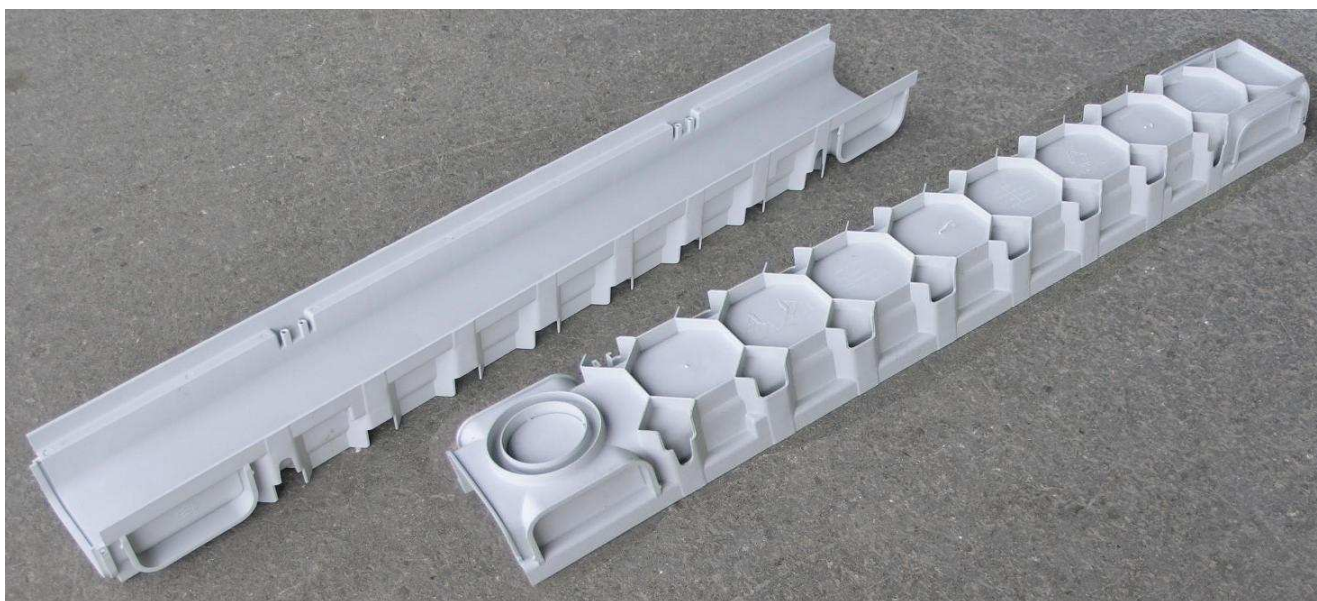
žlábek PEGASUS PLUS se nyní vyrábí v rozměru 130 x 75 x 1000 mm
